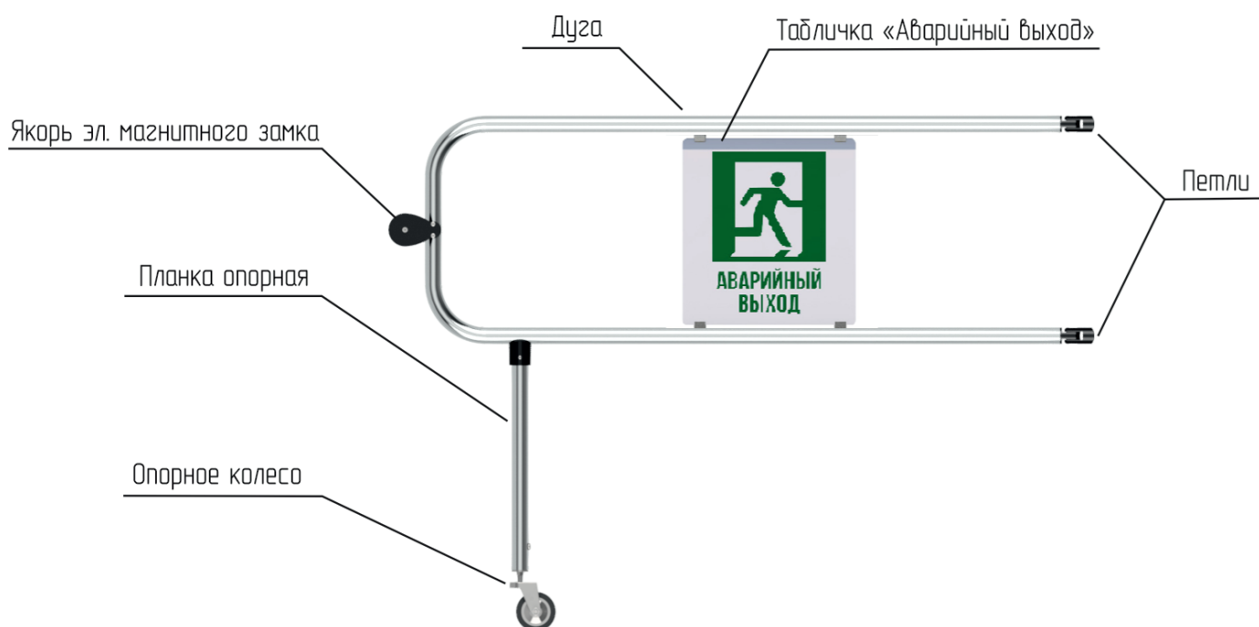
Рисунок 6.2.1 Створка «ХТА-02»
