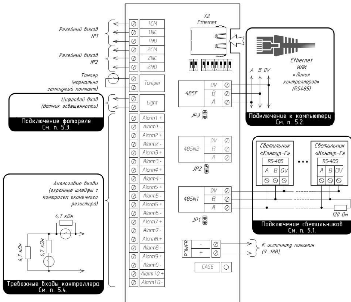
Рисунок 4. Обобщенная схема подключения контроллера «КЛ-Контур-С»
