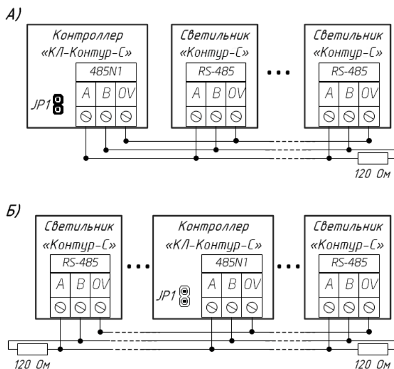
Рисунок 5. Подключение контроллера «КЛ-Контур-С» к «линии светильников» - А) контроллер первый (последний) в линии; Б) контроллер подключен посередине.
